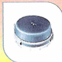
мина
